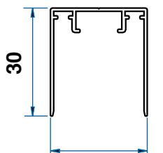
27 Guida superiore
