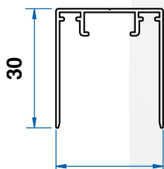
27 Guida superiore
