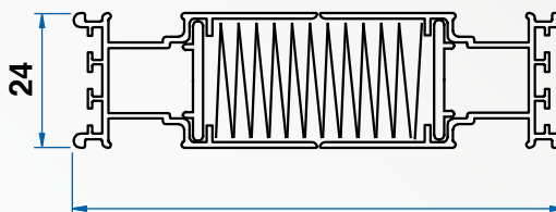
86 Profilo portarete
